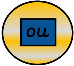
Jupiter
